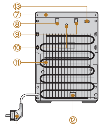
<후면>
